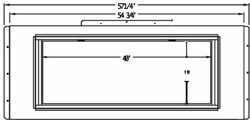
ELEVACION FRONTAL
